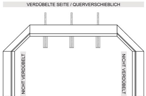
U-Sonderkonstruktion mit Con KS KW 170+ Frontteil (gerader Fugenverlauf)
