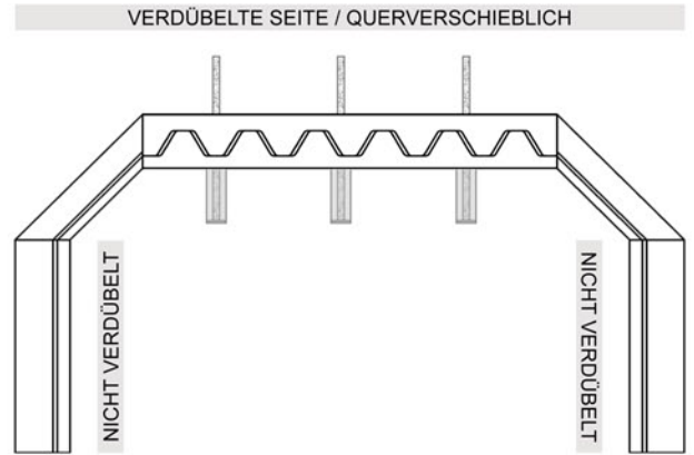
U-Sonderkonstruktion mit Con KS KW 170+ Trapez Frontteil
